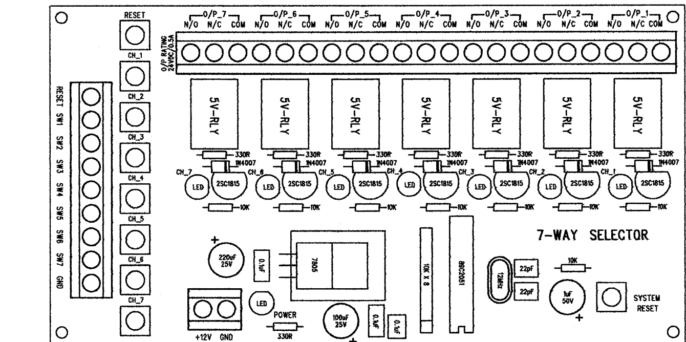
裝配圖
