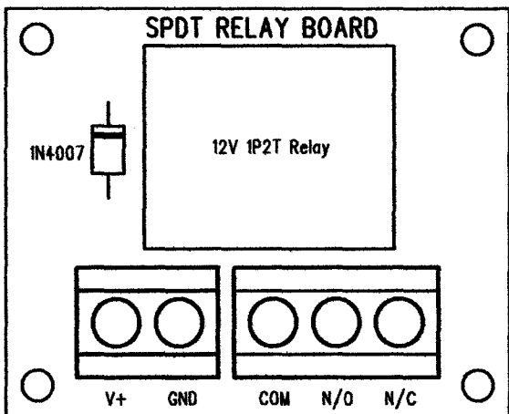
裝配圖
