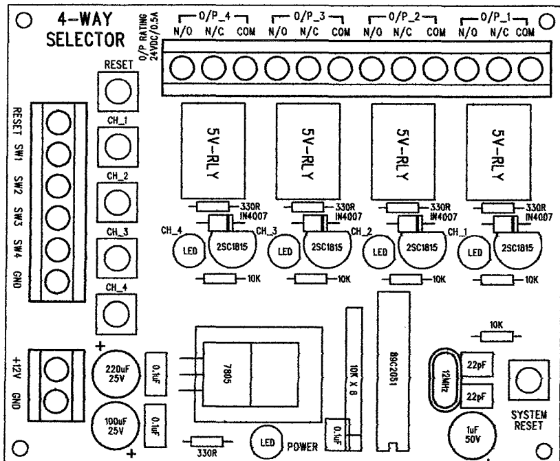
裝配圖
