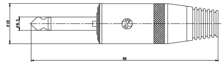
出线孔 \Phi 9
