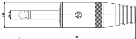
出线孔 \Phi 9
