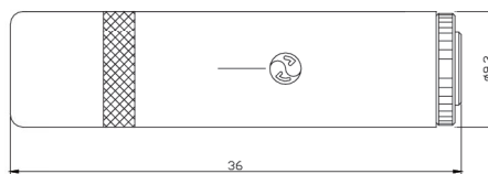
出线孔 \Phi 4.5
